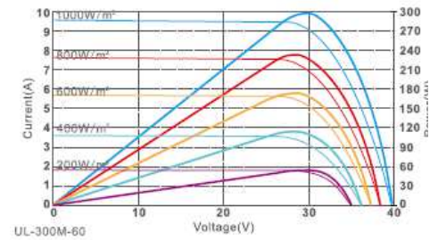
I-V charakterystyka
